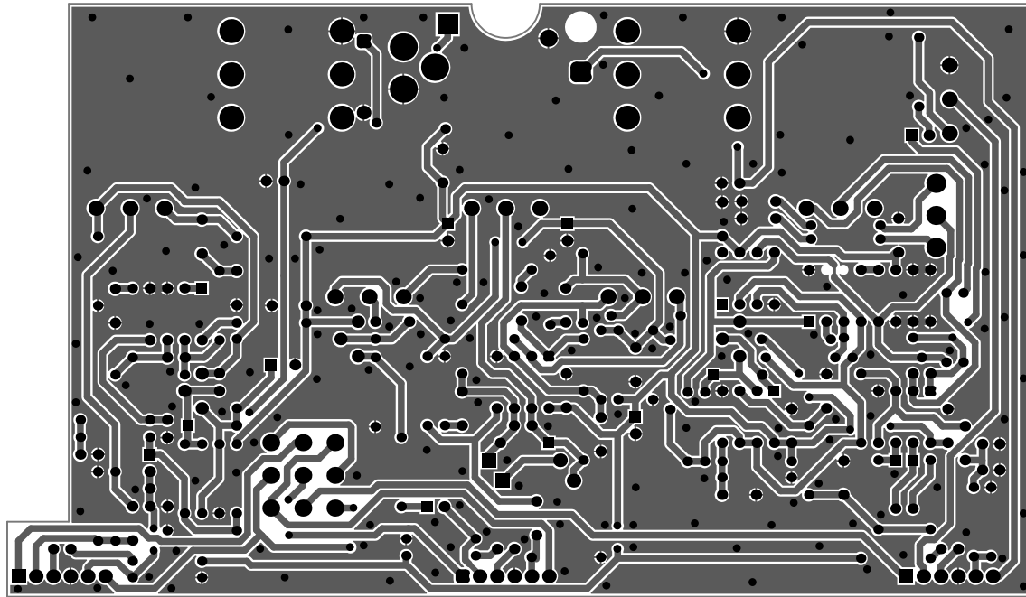
Cara Soldaduras
